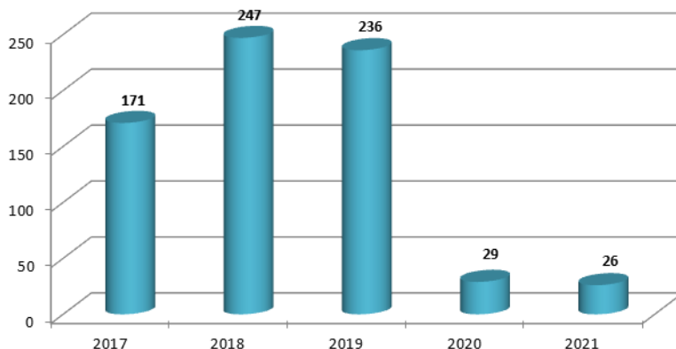
Количество дел об административных правонарушениях по ст.158 КоАП РК с 2017 по 2021 гг.
