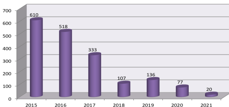
Количество дел по которым досудебное расследование прекращено с 2015-2021 гг.
